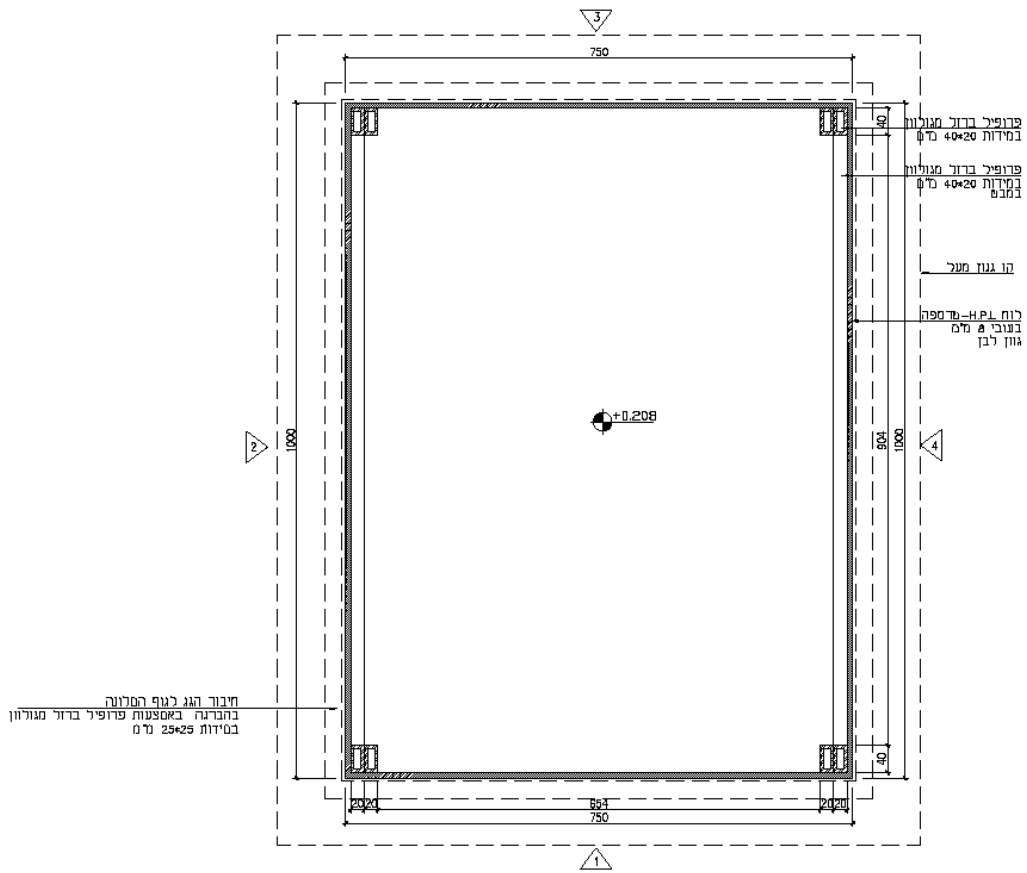
תכנית קנ"מ 1:5
