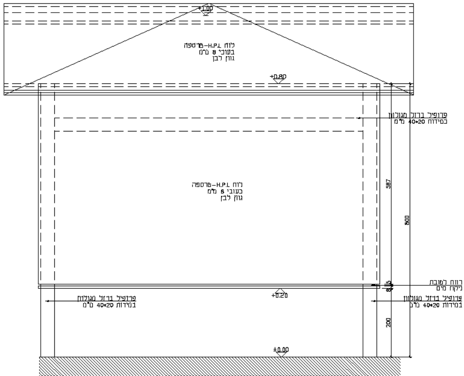
חבט 2 (גב) קנ"מ 1:5
